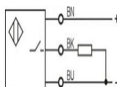
PNP NO
